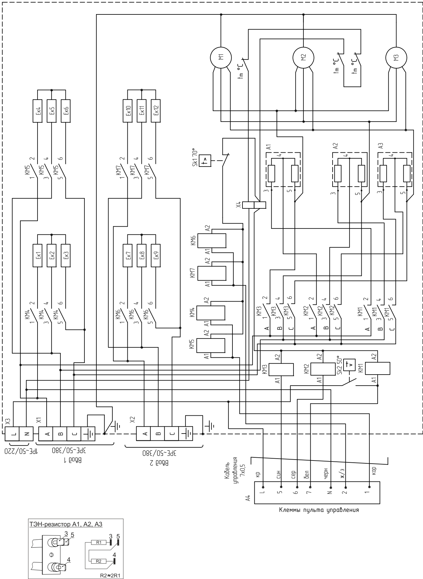
Рисунок 9. Электрическая схема занавесы КЭВ-36П7020Е
