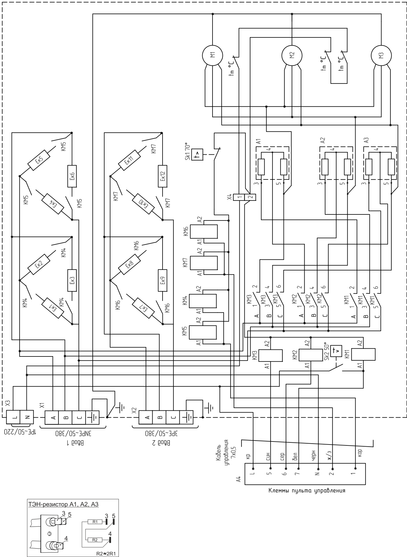
Рисунок 11. Электрическая схема занавесы КЭВ-60П7020Е
