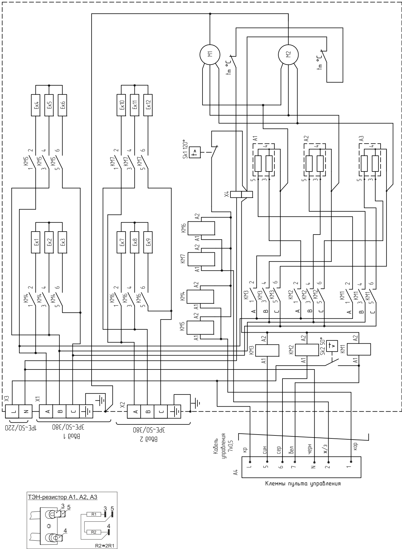
Рисунок 7. Электрическая схема занавесы КЭВ-24П7010Е и КЭВ-36П7010
