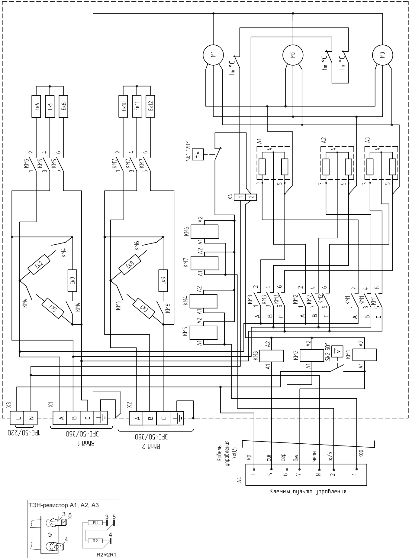
Рисунок 10. Электрическая схема занавесы КЭВ-48П7020Е
